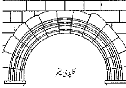
شکل 5a ایک پچی محراب میں کلیدی پتھر بالائی عمارت کے بوجھ کو محراب کی بنیاد منتقل کرتا ہے۔
