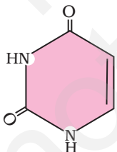
यूरेसील (पीरिमिडीन)
