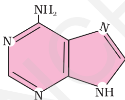
एडेनिन (प्यूरिन)
