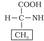
एलेनीन
