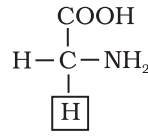
ग्लाइसीन
