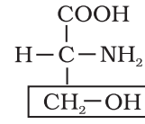
सीरीन
